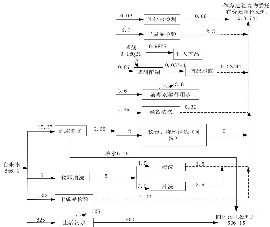
图 2-8 现有项目水平衡图 (单位 t/a)
