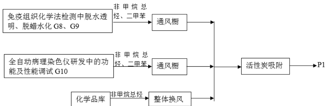
图 4-1 本项目有机废气处理流程示意图
