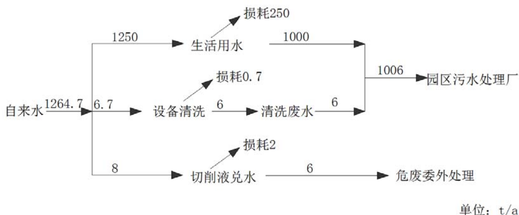
图 5-5 扩建后全厂水平衡图
