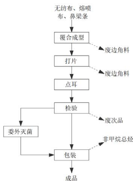
图 5-2 口罩生产工艺流程图
