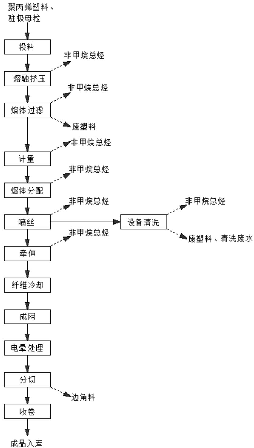
图 5-1 产业用纺织制成品（熔喷布）生产工艺流程图
