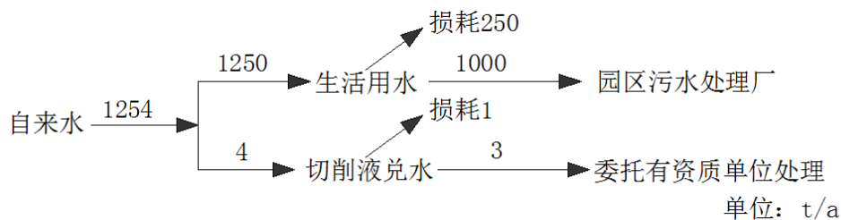
图 1-2 现有项目水平衡图
