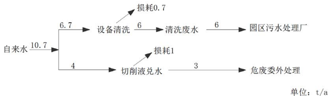
图 5-4 本项目水平衡图
