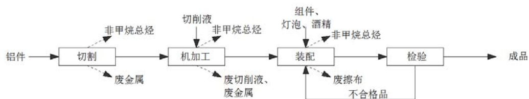
图 5-3 医用光学仪器生产工艺流程图
