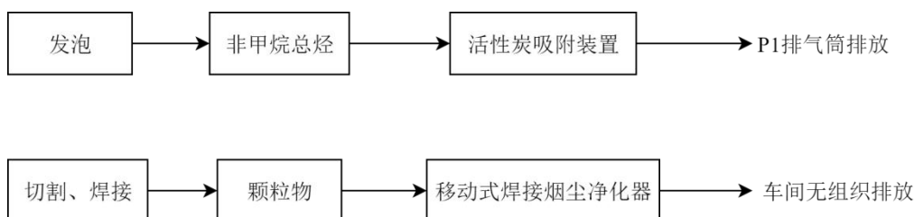
图 7-1 废气处理流程图
