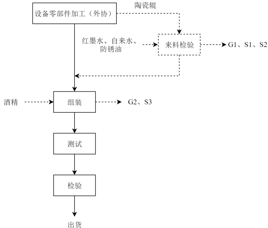
图 5-1 粉体设备工艺流程图
