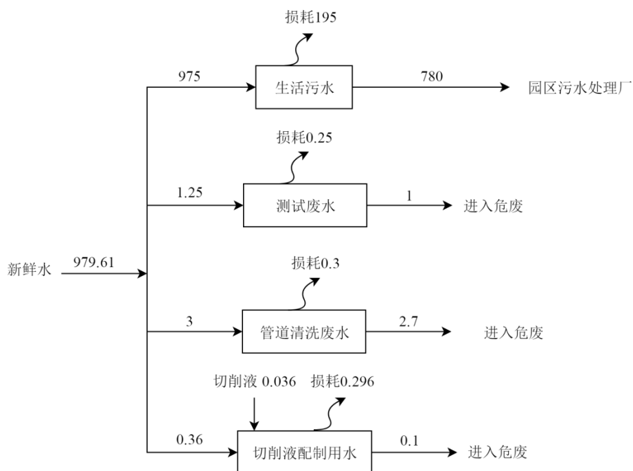
图 5-3 本项目水平衡图 (t/a)
