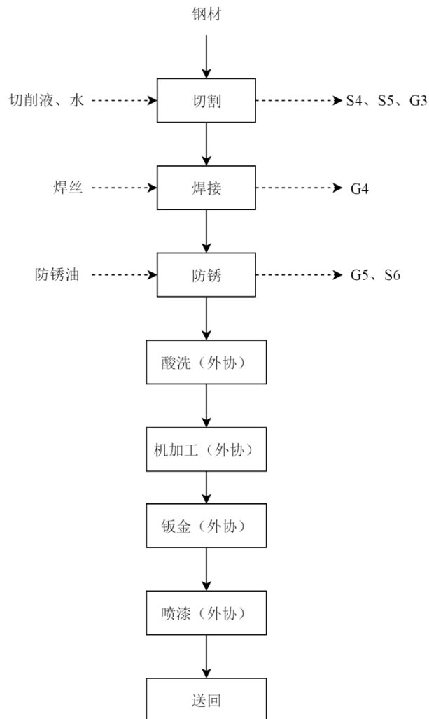
图 5-2 陶瓷对辊破碎机架台工艺流程图
